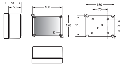
Elektroinstalační krabice IP55 - Obj.č. / Item 3042
