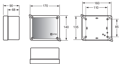
Elektroinstalační krabice IP55 - Obj.č. / Item 3043
