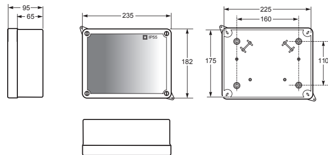
Elektroinstalační krabice IP55 - Obj.č. / Item 3045
